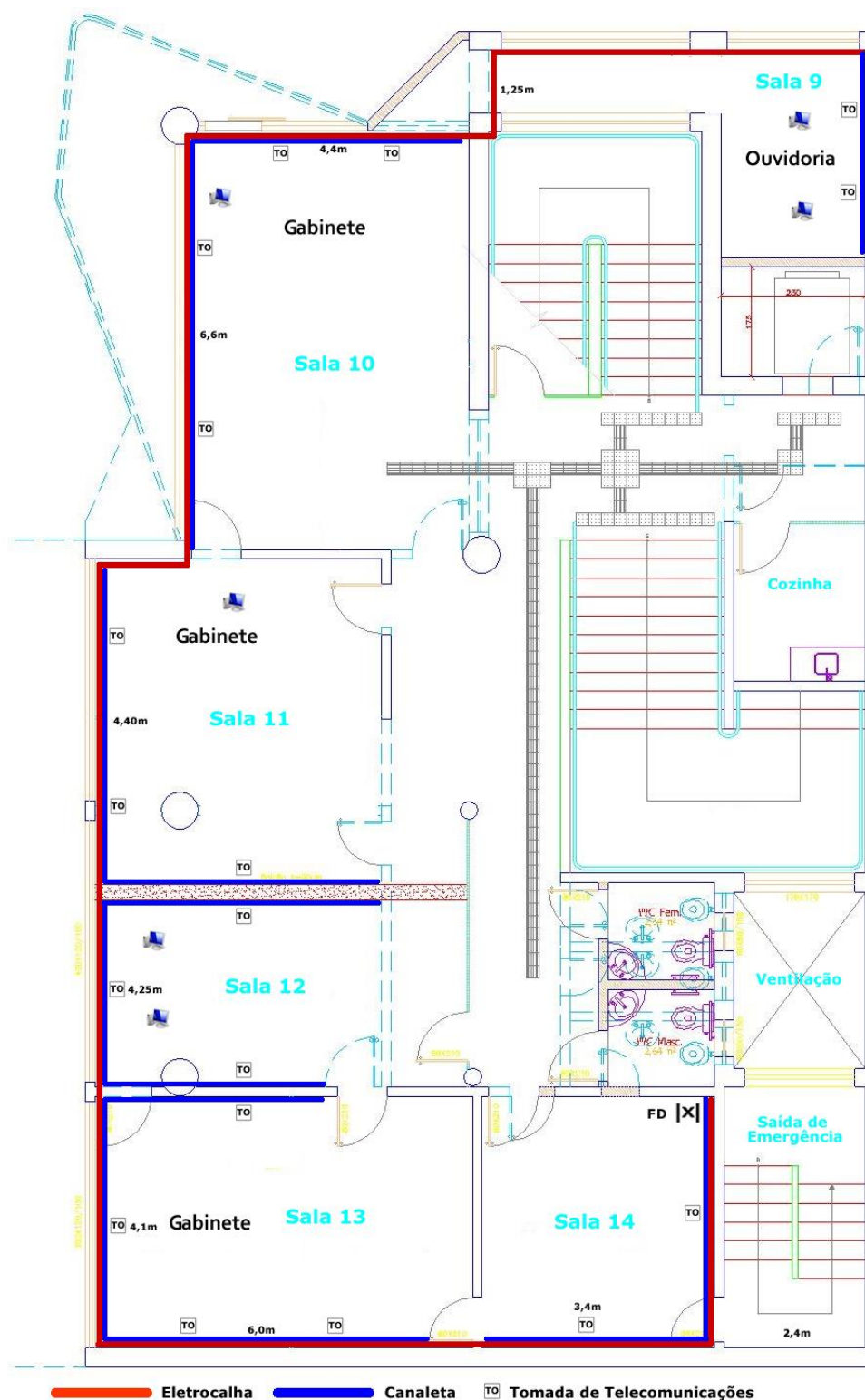
Figura 4 – Planta baixa do pavimento 2
