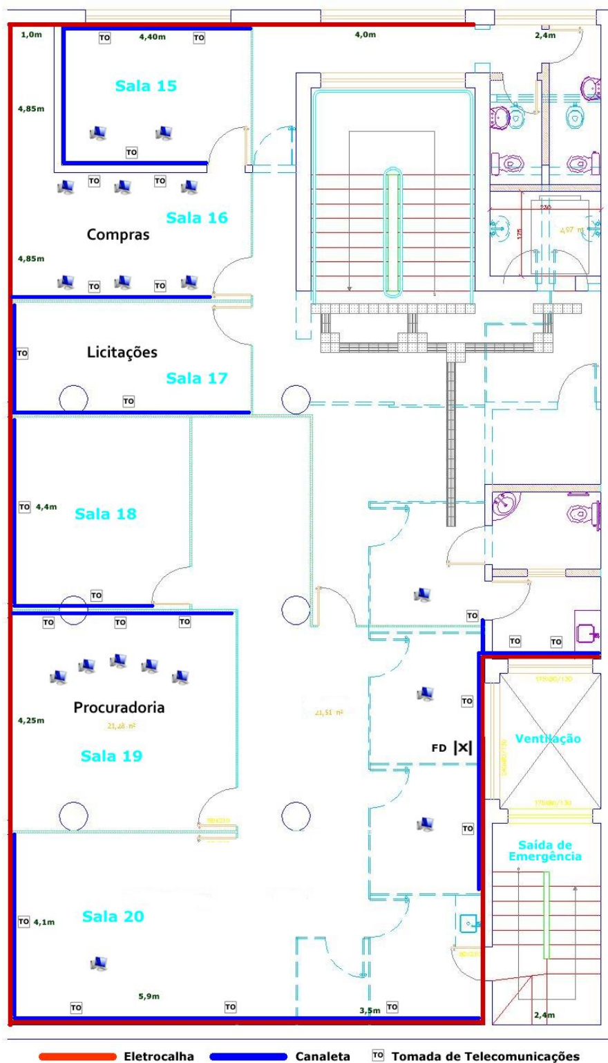
Figura 5 – Planta baixa do pavimento 3
