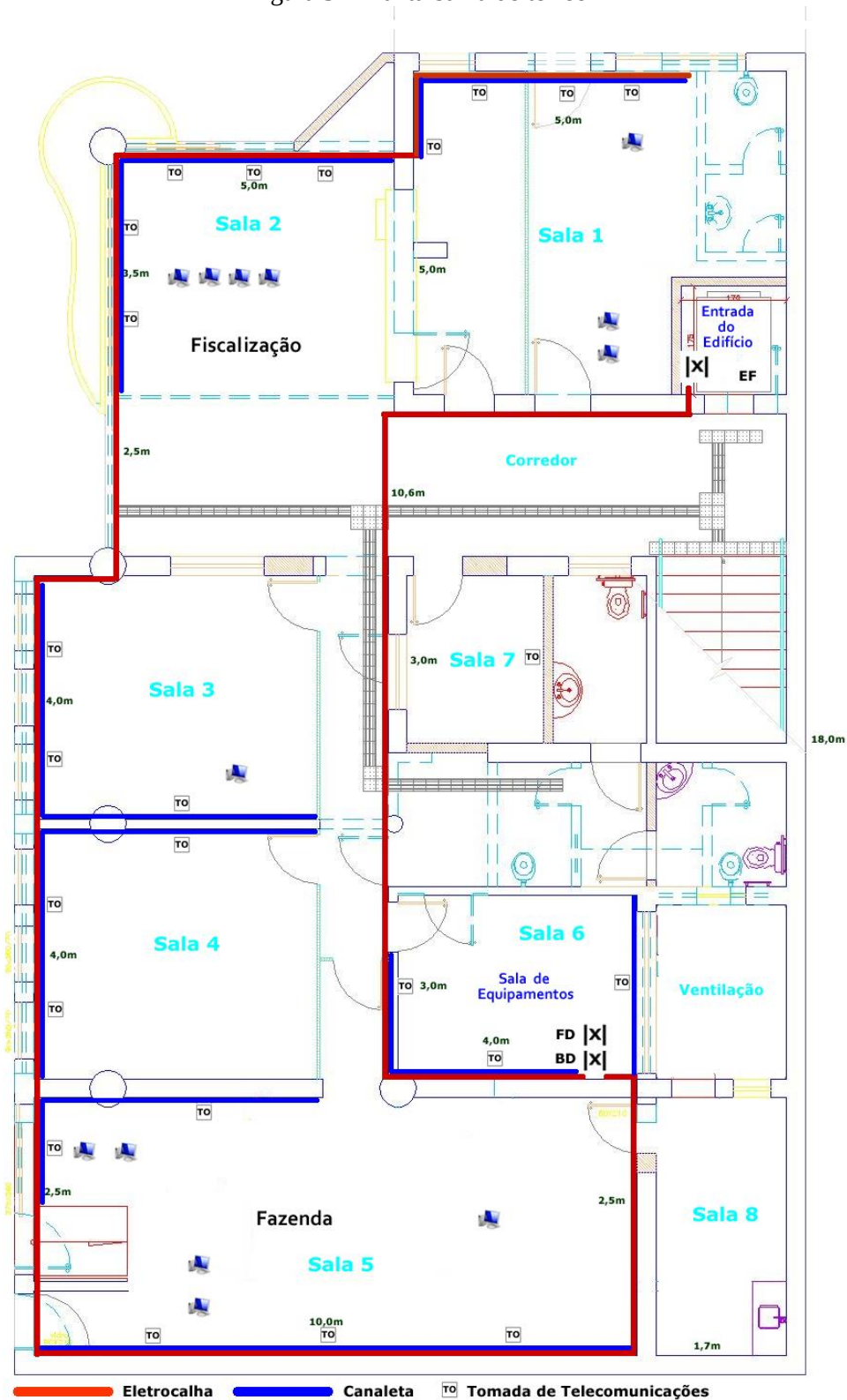
Figura 3 – Planta baixa do térreo
